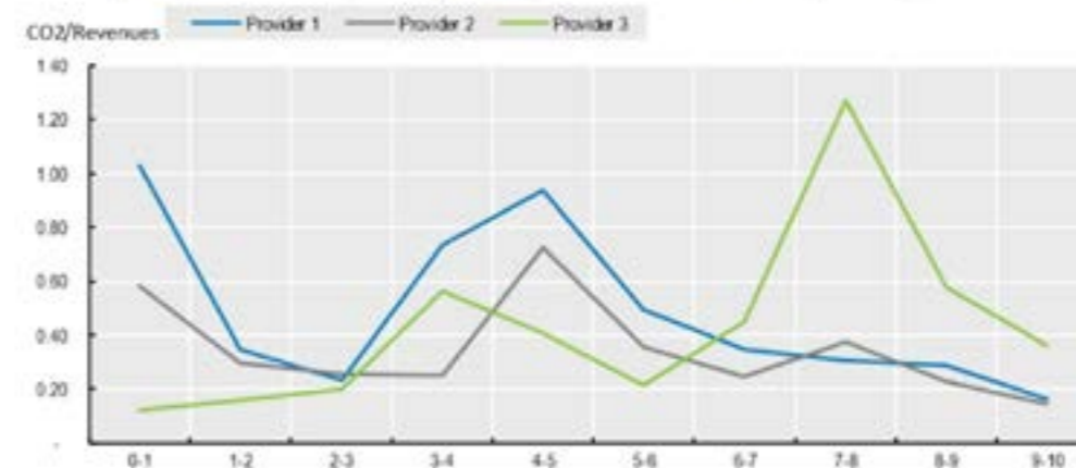
Gráfico 3. Emisiones de CO2 y evaluación de acuerdo al pilar ambiental de ESG de un conjunto global de compañías, ajustado por tamaño de las compañías según ventas
