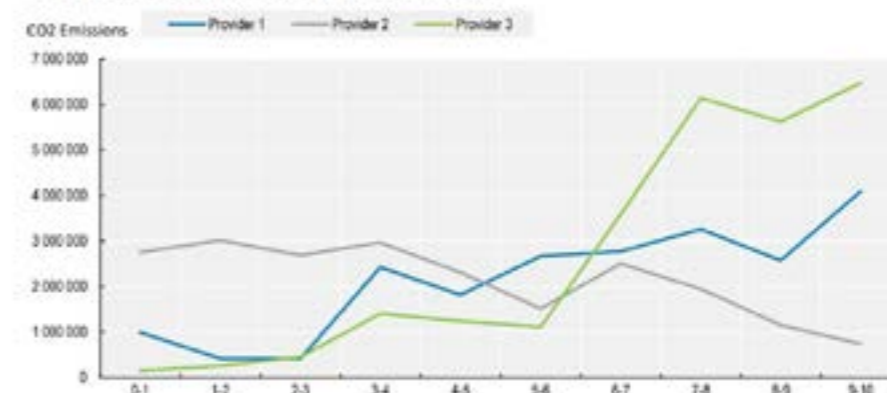
Gráfico 2. Emisiones de CO2 y evaluación de acuerdo al pilar ambiental de ESG de un conjunto global de compañías
